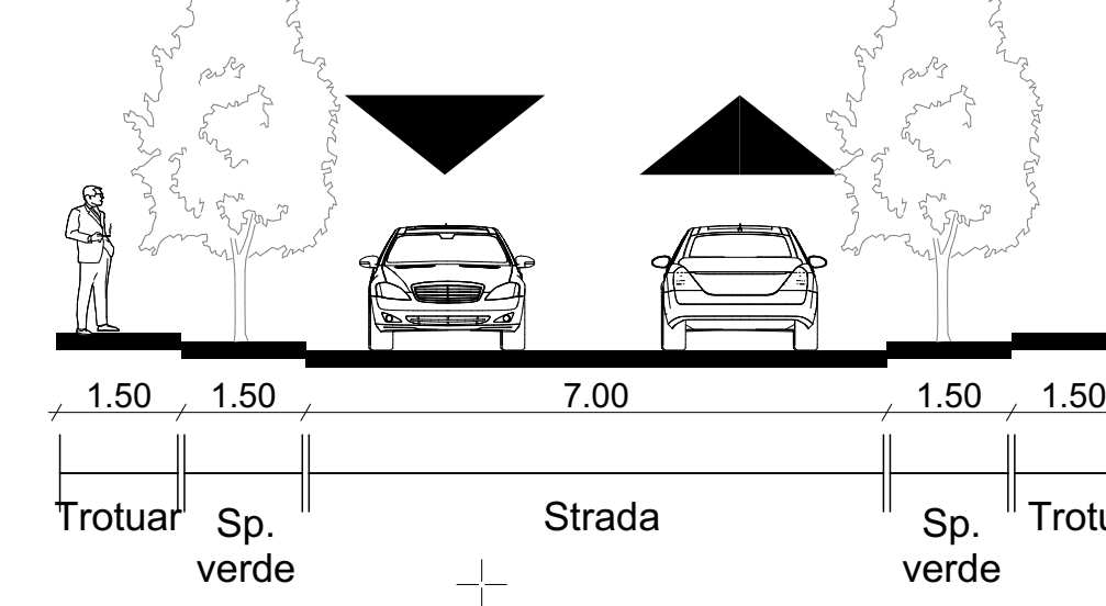
Profil transversal Str. Tazlului Sc 1/100
